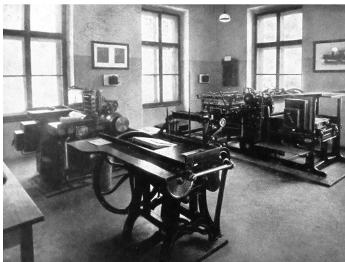
Příloha 19: Strojovna odborné pokračovací školy (PETLAN, Odborná škola , obr. 3).
