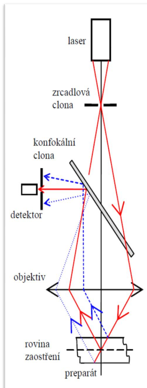
Obrázek 11: Schéma skenovacího mikroskopu
