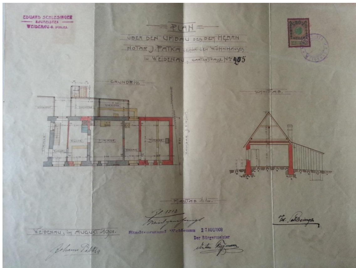
Plán č. 1 Plán přestavby domu Johanna Patky, notáře ve Vidnavě (Převzato s laskavým svolením SOkA Jeseník, Fond Archiv města Vidnava (1291) 1408 – 1945 (1948), inv. č. 950, plán č. 24)
