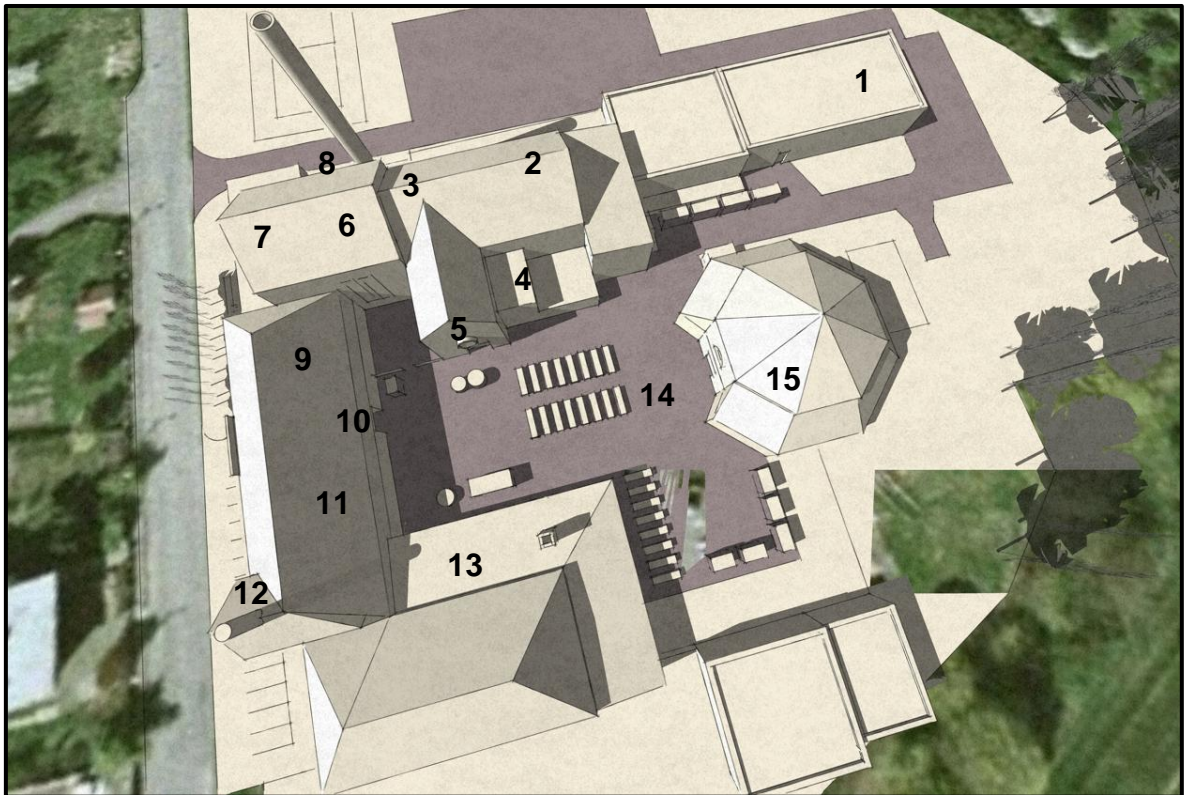
Obrázek 1: Plánek areálu pivovaru v Kostelci nad Černými lesy: 1 - dílny, 2 - chladicí štoky, spilky, ležácké sklepy, lednice, 3 - varna a nadvarní, 4 - sprchový aparát, 5 - výtah, 6 - strojovna, 7 - kompresorovna, 8 - komín, 9 - zájezdní hostinec, 10 - průjezd, 11 - malé sladovnické humno, 12 - sladovnický hvozď, 13 - velké sladovnické humno, 14 - pivovarský dvůr, 15 - žentourový mlýn.
