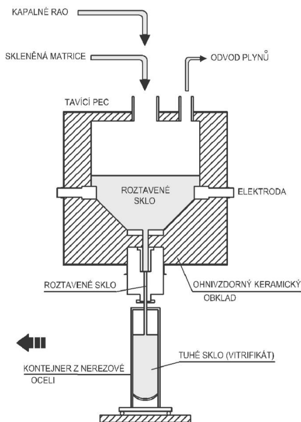
Obr. 3.1 Jednostupňová tavící pec [Převzato z [6]]
