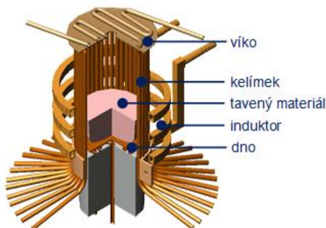
Obr. 4.1 Schéma studeného kelímku [Převzato z [24]]
