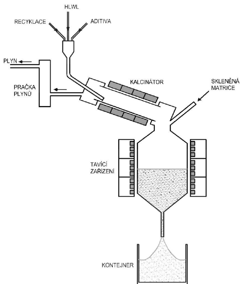
Obr. 3.2 Princip dvoustupňové vitrifikace [Převzato z [6]]
