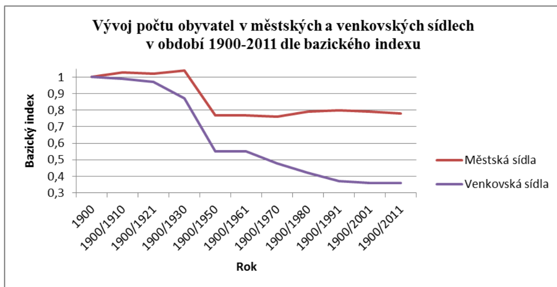
Graf číslo 7: Vývoj počtu obyvatel v městských a venkovských sídlech v období 1900-2011 dle bazického indexu
