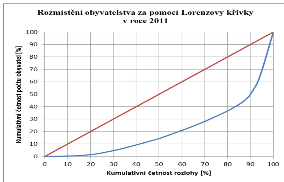
Graf číslo 5: Rozmístění obyvatelstva za pomoci Lorenzovy Křivky v roce 2011
