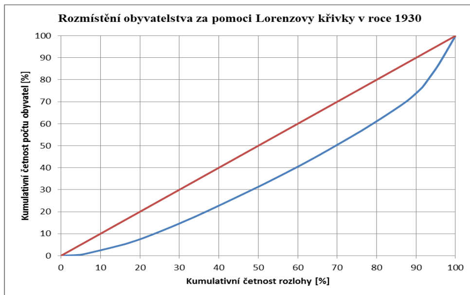
Graf číslo 3: Rozmístění obyvatelstva za pomoci Lorenzovy Křivky v roce 1930
