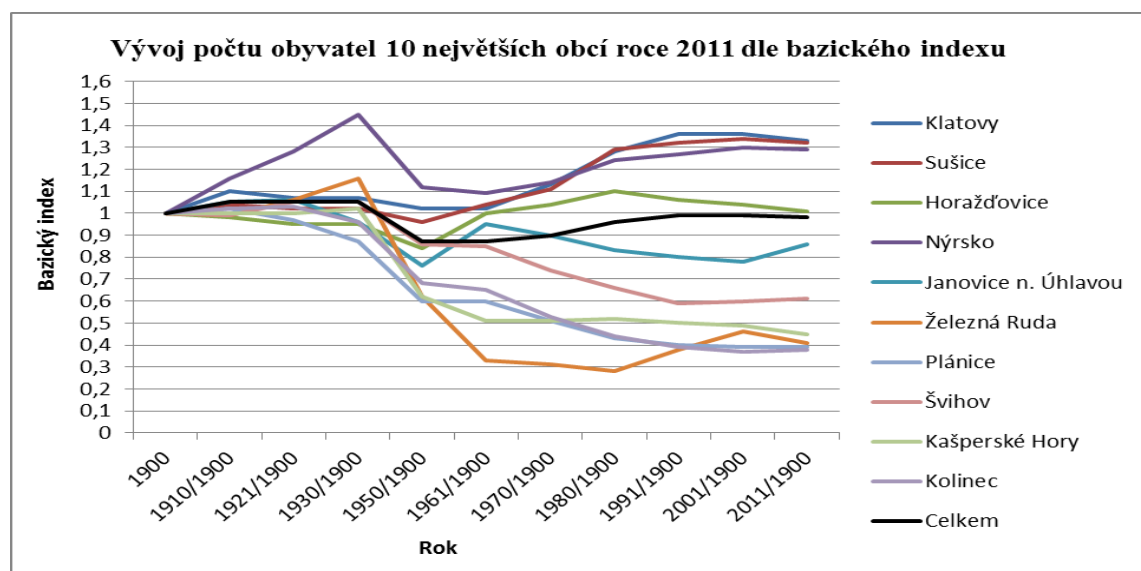
Graf číslo 6: Vývoj počtu obyvatel 10 největších obcí roce 2011 dle bazického indexu
