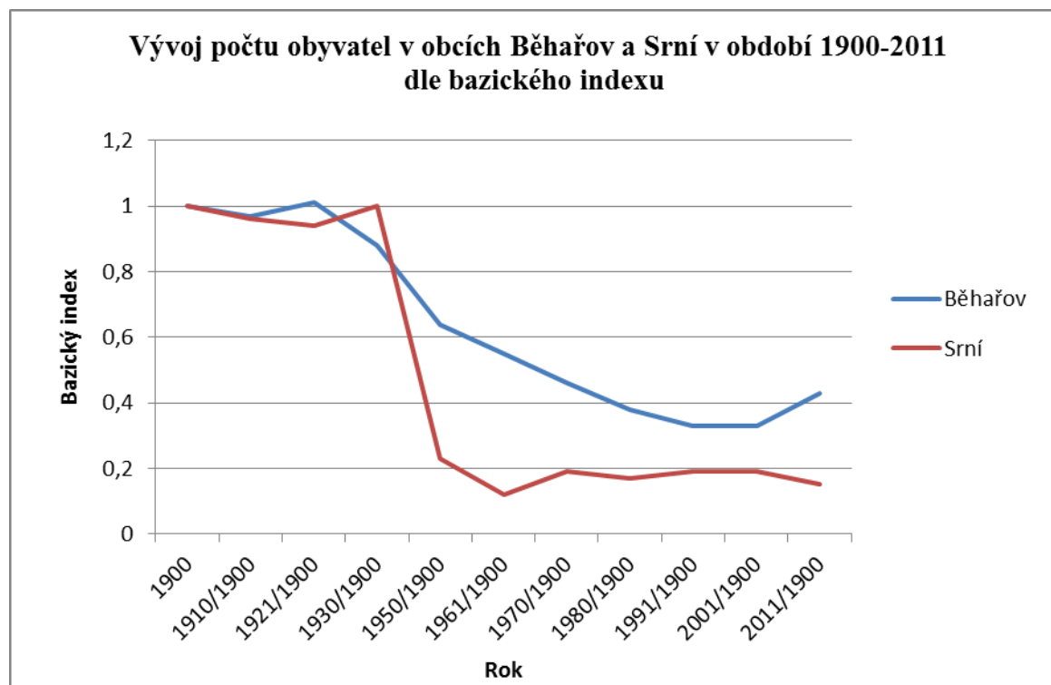
Graf číslo 8 Vývoj počtu obyvatel v obcích Běhařov a Srní v období 1900-2011 dle bazického indexu
