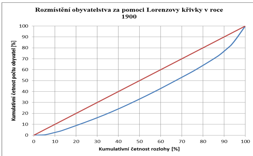
Graf číslo 2: Rozmístění obyvatelstva za pomoci Lorenzovy Křivky v roce 1900
