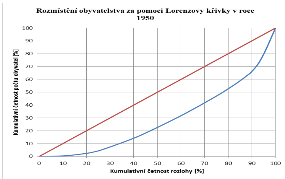
Graf číslo 4: Rozmístění obyvatelstva za pomoci Lorenzovy Křivky v roce 1950
