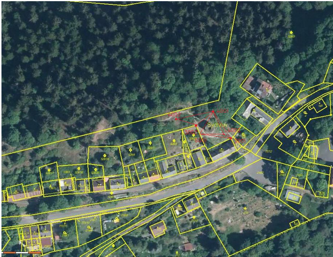
Obr. 13: Model vytyčeného zaměřovacího polygonu na lokalitě.
