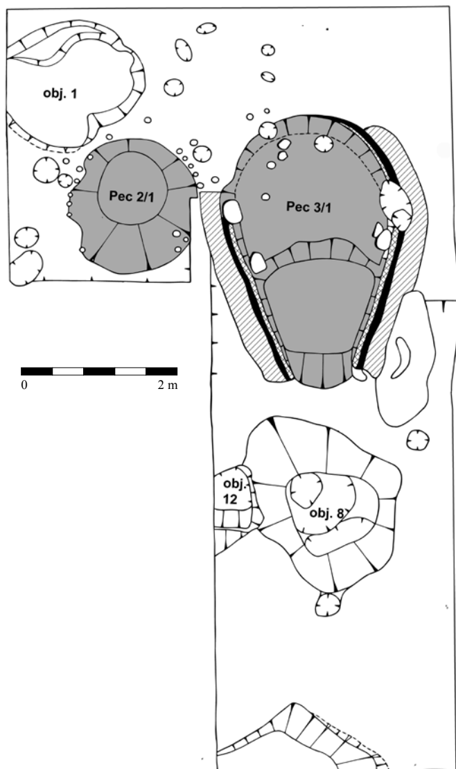
Obr. 9. Hrnčířská pec z České Lípy – pece č. 2/1 a 3/1 vyznačeny. Podle Gabriel 1979, obr. 1, upravil L. Čapek. Abb. 9. Töpferofen aus Česká Lípa – Öfen Nr. 2/1 und 3/1 gekennzeichnet. Nach Gabriel 1979, Abb. 1, bearbeitet von L. Čapek.
