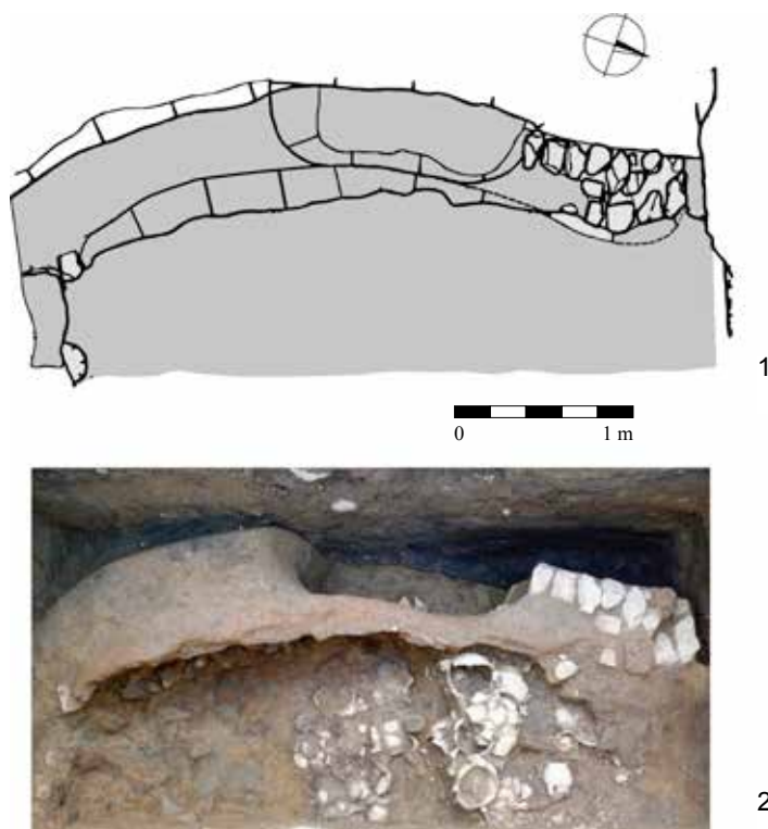
Obr. 18. Hrnčířská pec (s. j. 8-034) z Berouna – Hořejšího předměstí. 1 – půdorys, 2 – fotografie pece včetně keramické klenby. Podle Vyšohlíd 2015a, obr. 6 a 7, upravil L. Čapek.
