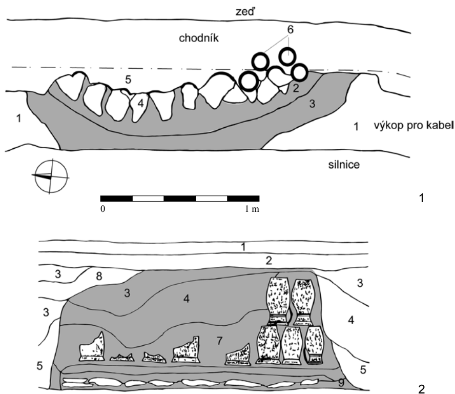
Obr. 14. Hrnčířská pec z Horšovského Týna. 1 – půdorys pece na hraně výkopu, 2 – řez stěnami pece včetně umístění keramických nádob; popis uložení: 1 – chodník z dlaždic, 2 – vyrovnávací štěrkopísková navážka, 3 – destrukční vrstva pece, 4 – mazanice se zlomky nádob, 5 – žlutka, uhlíky, zlomky keramiky, 6 – jílovité podloží, 7 – keramika uložená v mazanici, 8 – hlinito-písčité vrstva s obsahem zlomkové keramiky, 9 – přepálená žlutka s kameny základu pece. Podle Frýda 1992, Tab. IV a V, upravil L. Čapek.
