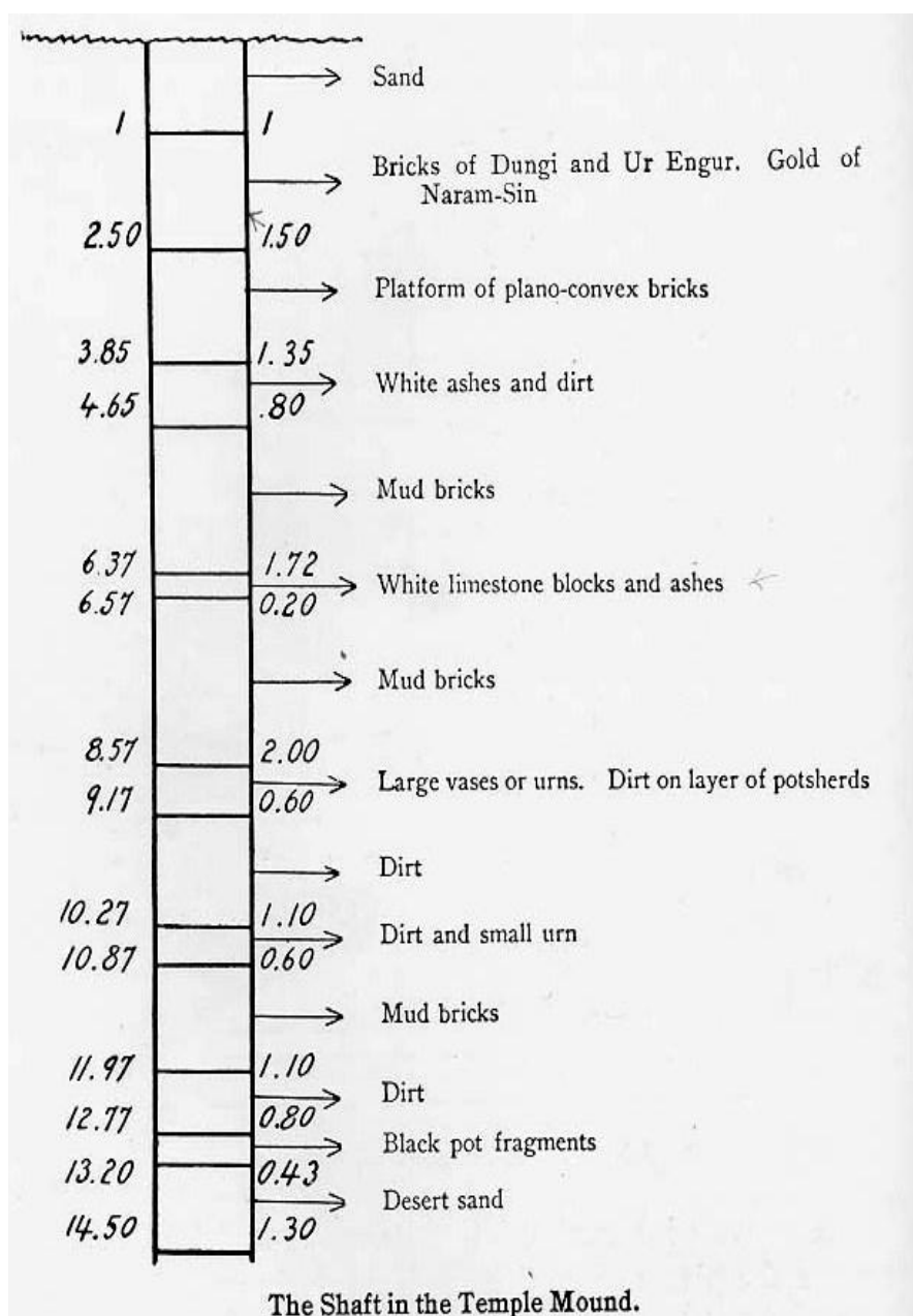
Obrázek 9: Jihozápadní šachta pahorku V.
