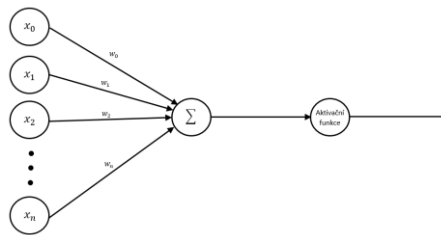
Obr. 4) Perceptron
