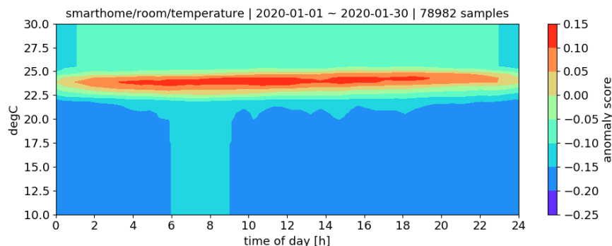
OBRÁZEK A1.4: Graf popisující získané skóre pomocí klasifikace z natrénovaného modelu pro vnitřní teplotu
