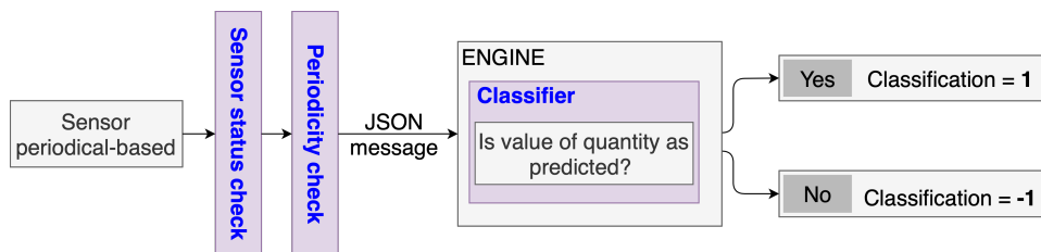
OBRÁZEK 4.9: Výstupy subsystému klasifikace z natrénovaného modelu u 2D veličin
