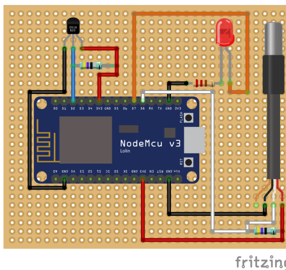
OBRÁZEK 2.6: Schéma obvodu platformy NodeMCU, dvou čidel DS18B20 a led diody na plošném spoji
