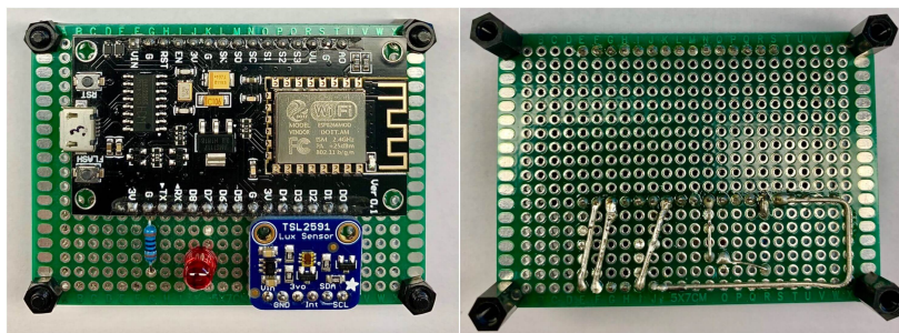
OBRÁZEK 2.10: Fyzická realizace senzoru s modulem TSL2591
