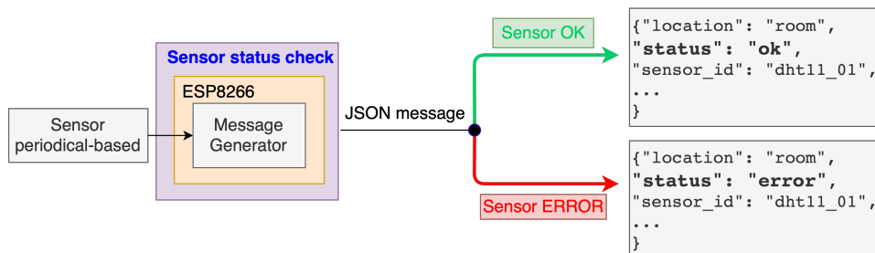
OBRÁZEK 4.4: Výstupy subsystému detekce chyb na úrovni mikročipu ESP8266
