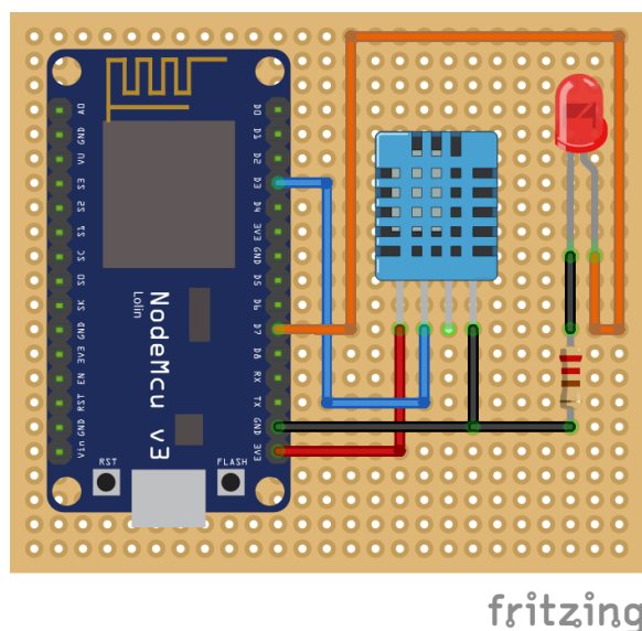
OBRÁZEK 2.8: Schéma obvodu platformy NodeMCU, modulu DHT11 a led diody na plošném spoji
