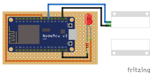
OBRÁZEK 2.15: Schéma obvodu platformy NodeMCU, magnetického kontaktu LS311B38 a led diody na plošném spoji
