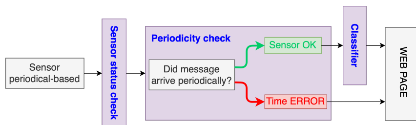
OBRÁZEK 4.6: Výstupy subsystému kontroly periodicity příchozích zpráv
