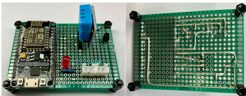
OBRÁZEK 2.7: Fyzická realizace senzoru s moduly DS18B20 a DHT11
