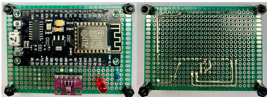
OBRÁZEK 2.12: Fyzická realizace senzoru s modulem BME280
