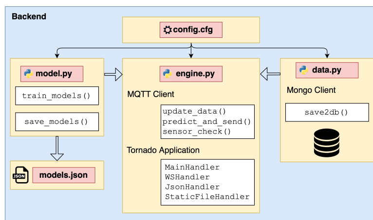
OBRÁZEK 3.4: Diagram architektury kódu backendu na Raspberry Pi
