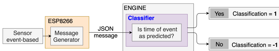
OBRÁZEK 4.7: Výstupy subsystému klasifikace z natrénovaného modelu u 1D veličin
