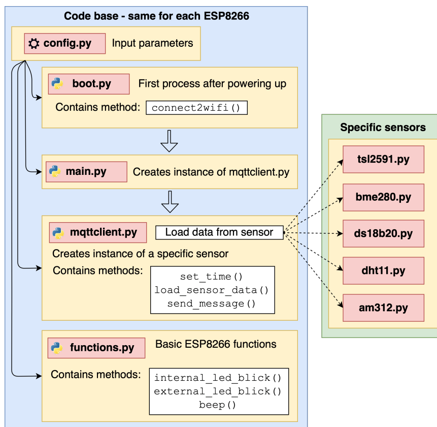
OBRÁZEK 2.5: Diagram architektury kódu na mikročipu ESP8266
