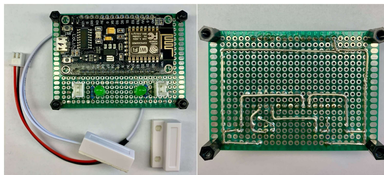
OBRÁZEK 2.16: Fyzická realizace senzoru s magnetickým kontaktem LS311B38
