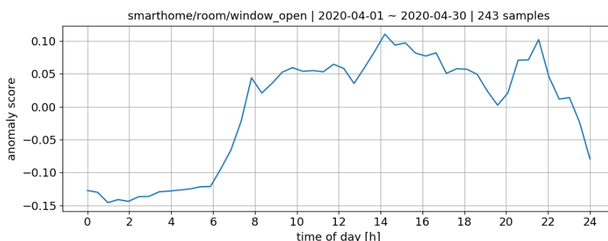
OBRÁZEK 4.8: Graf popisující získané skóre pomocí klasifikace z natrénovaného modelu pro status okna
