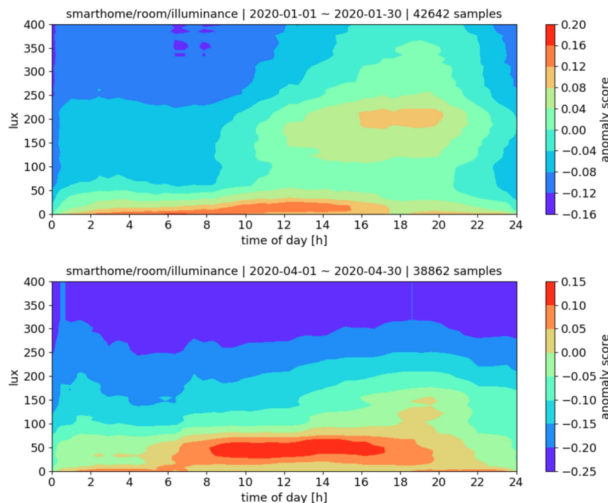
OBRÁZEK 4.10: Graf popisující získané skóre pomocí klasifikace z natrénovaného modelu pro intenzitu osvětlení v místnosti
