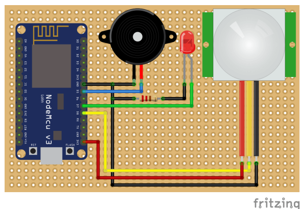
OBRÁZEK 2.13: Schéma obvodu platformy NodeMCU, modulu AM312, led diody a externího bzučáku na plošném spoji
