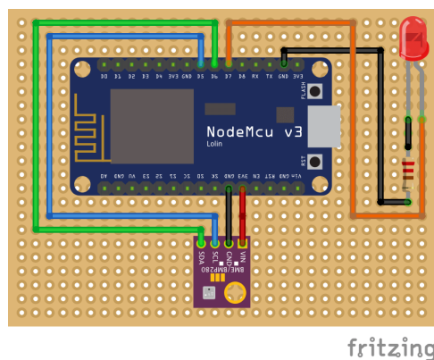
OBRÁZEK 2.11: Schéma obvodu platformy NodeMCU, modulu BME280 a led diody na plošném spoji
