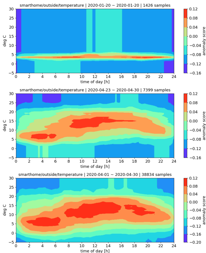
OBRÁZEK A1.3: Graf popisující získané skóre pomocí klasifikace z natrénovaného modelu pro venkovní teplotu
