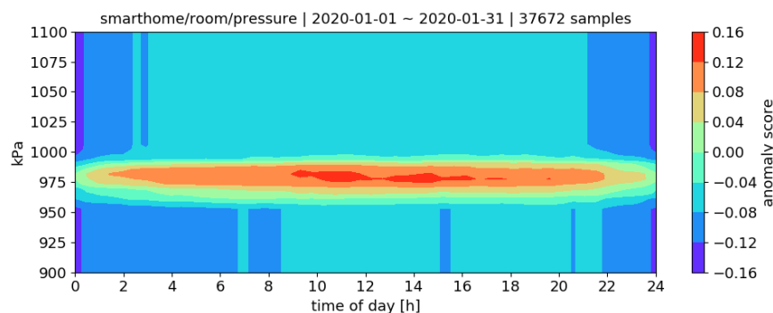
OBRÁZEK A1.5: Graf popisující získané skóre pomocí klasifikace z natrénovaného modelu pro intenzitu osvětlení v místnosti
