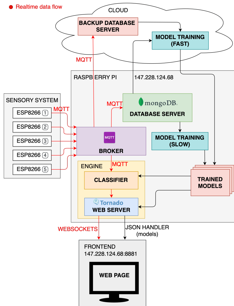
OBRÁZEK 3.1: Rozložení jednotlivých komponent a schéma datových toků v celém projektu
