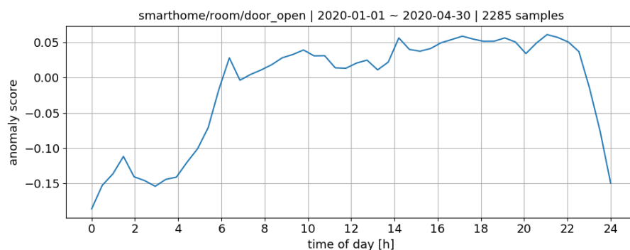
OBRÁZEK A1.1: Graf popisující získané skóre pomocí klasifikace z natrénovaného modelu pro status dveří
