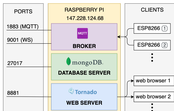
OBRÁZEK 3.3: Schéma procesů s popisy portů běžících na Raspberry Pi
