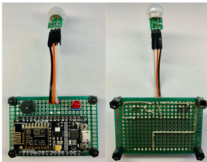
OBRÁZEK 2.14: Fyzická realizace senzoru s modulem AM312
