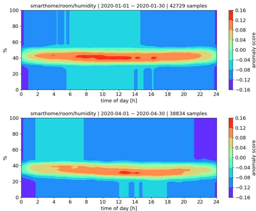
OBRÁZEK A1.6: Graf popisující získané skóre pomocí klasifikace z natrénovaného modelu pro vlhkost v místnosti
