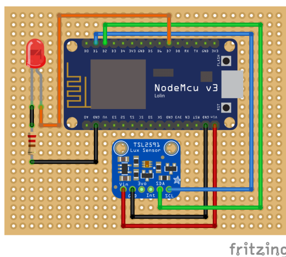
OBRÁZEK 2.9: Schéma obvodu platformy NodeMCU, modulu TSL2591 a led diody na plošném spoji
