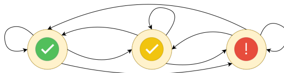
OBRÁZEK 4.3: Markovův řetězec popisující přechody mezi jednotlivými stavy senzorů
