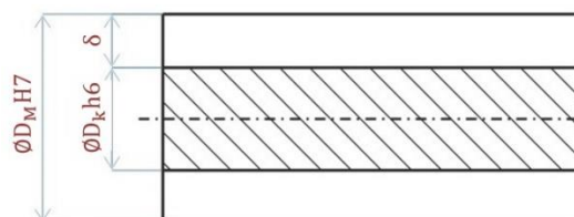
Obr. 4-4 – předepsané tolerance modelu a výměnných disků
