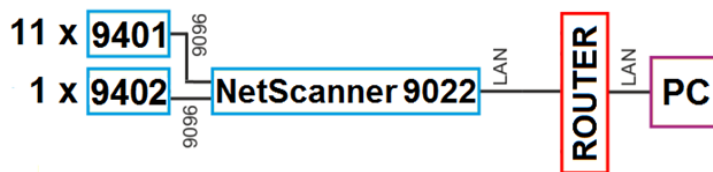
Obr. 4-9 – schéma měřicího řetězce tlaků
