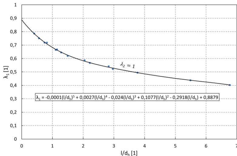
Obr. 5-30 – rychlostní poměry na vstupu do štěrbin při \lambda_2 = 1
