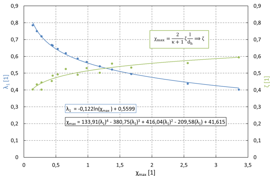
Obr. 5-32 – závislost bezrozměrné vstupní rychlosti \lambda_1 a ztrátového součinitele \zeta na poměrné délce štěrbin
