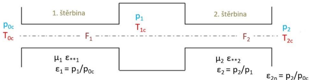
Obr. 3-3 – výpočtové schéma průtočného systému štěrbin
