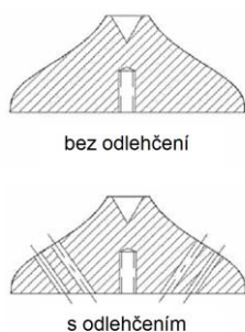
Obr. 2-9 – profilovaná kuželka bez odlehčení a s odlehčením [35]
