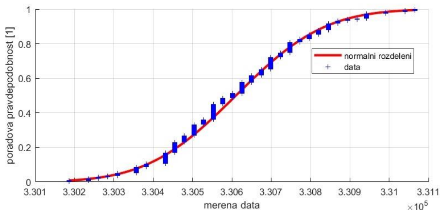
Obr. 4-16 – odhad kumulativní distribuční funkce
