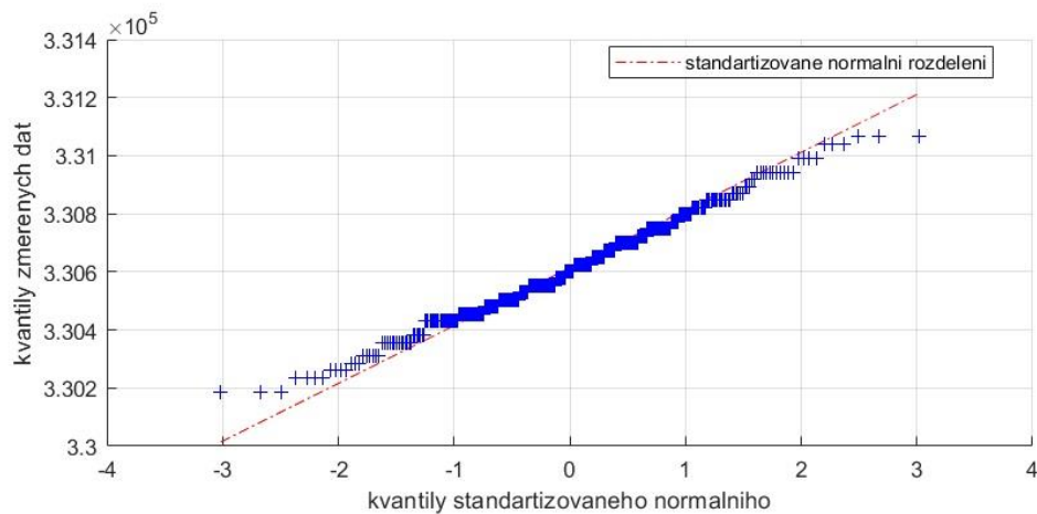
Obr. 4-17 – Q-Q graf – porovnání se standardizovaným normálním rozdělením
