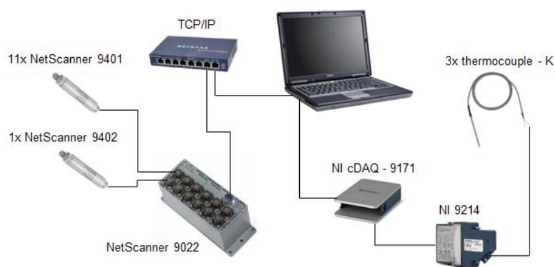
Obr. 4-5 – schéma zapojení měřících přístrojů
