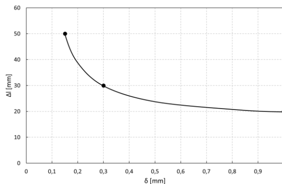
Obr. 5-22 – závislost \Delta l na \delta
