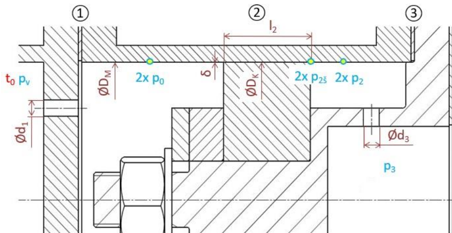
Obr. 4-3 – detailní provedení modelu štěrbin
