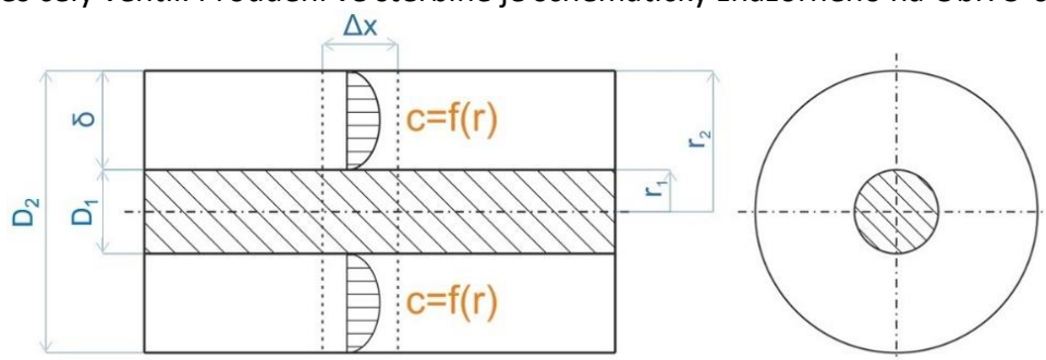
Obr. 3-6 – proudění ve štěrbině
