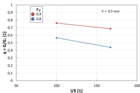
Obr. 5-18 – závislost poměrného hmotnostního průtoku q na poměrné délky štěrbinu
