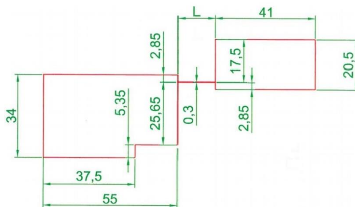
Obr. 2-14 – schéma výpočtové oblasti [19]
