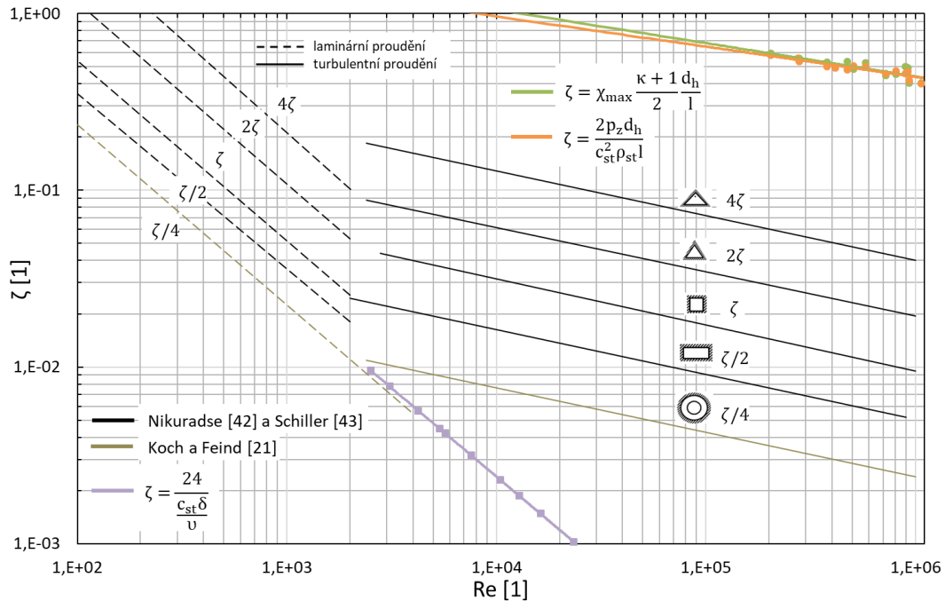
Obr. 5-33 – ztrátový součinitelé různě tvarovaných tvarů
