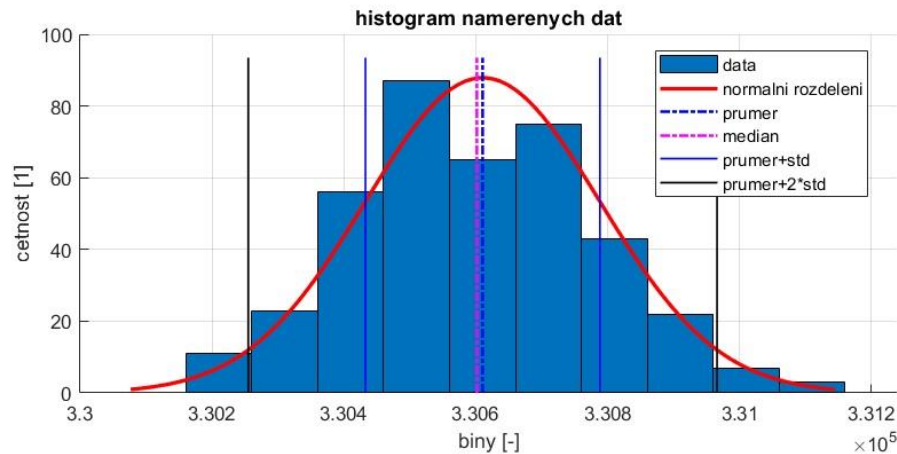
Obr. 4-13 – histogram měřeného tlaku p_{2l} – vyznačení základních statických parametrů
