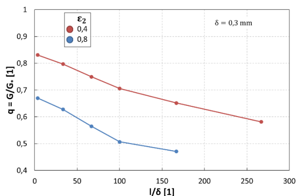
Obr. 5-16 – závislost poměrného hmotnostního průtoku q na poměrné délky štěrbinu
