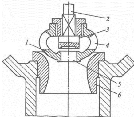
Obr. 1-2 – odlehčený ventil trámcové regulace MEI [2]
