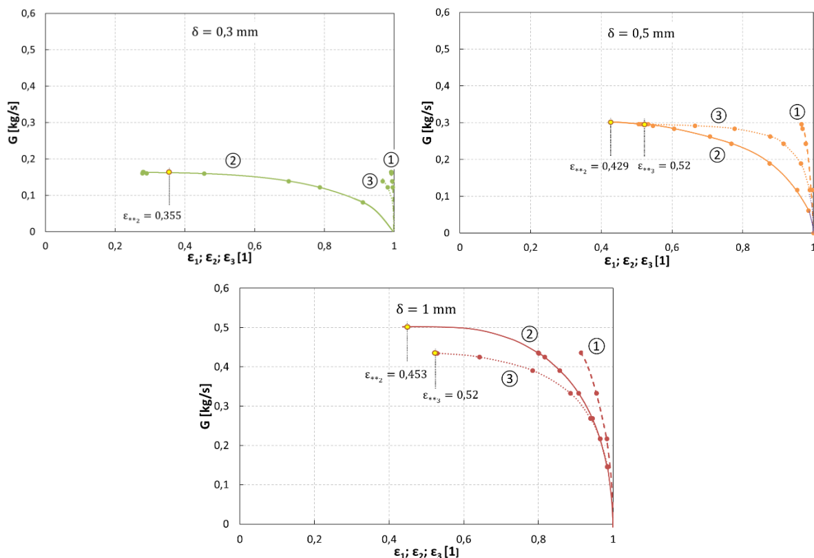
Obr. 5-1 – hmotnostní průtoky částmi odlehčovacího systému
