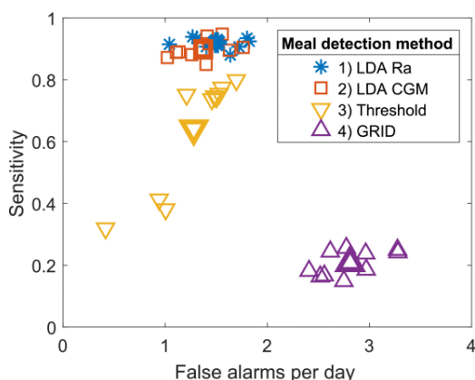
Obrázek 3.11: Úspěšnost detekce
