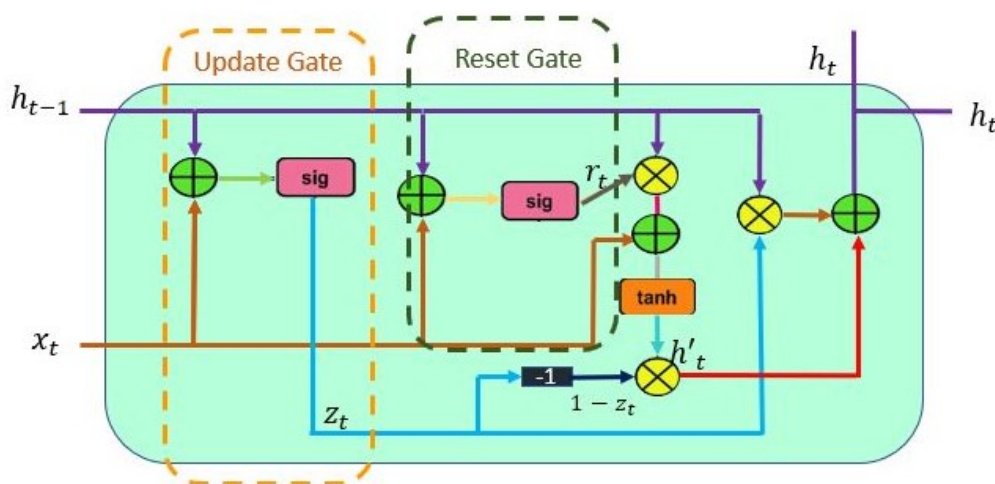
Obrázek 6.3: GRU buňka
