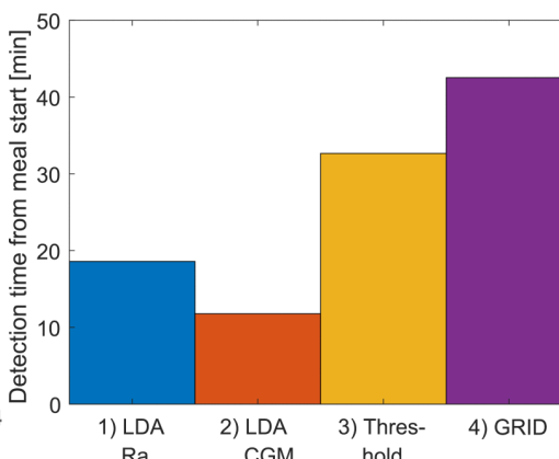
Obrázek 3.12: Zpoždění detekce
