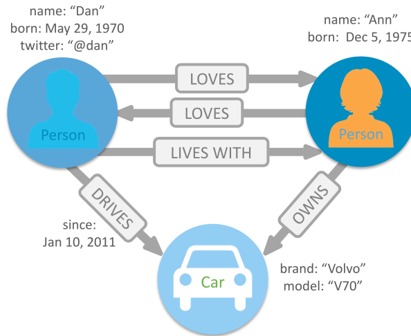
Obrázek 3.7: Ukázkou grafové databáze. Převzato z [19].
