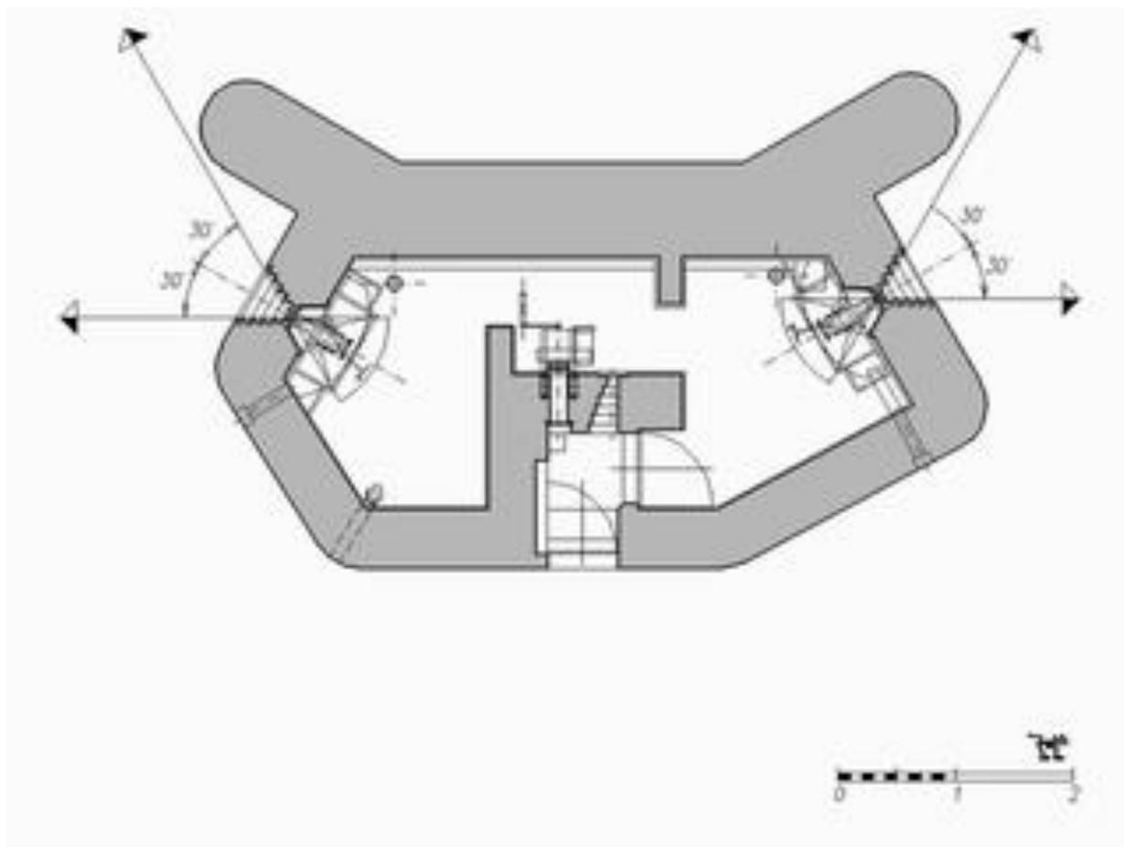
Obrázek 23 - Objekt D-31/79/A-120 (plánový nákres)
