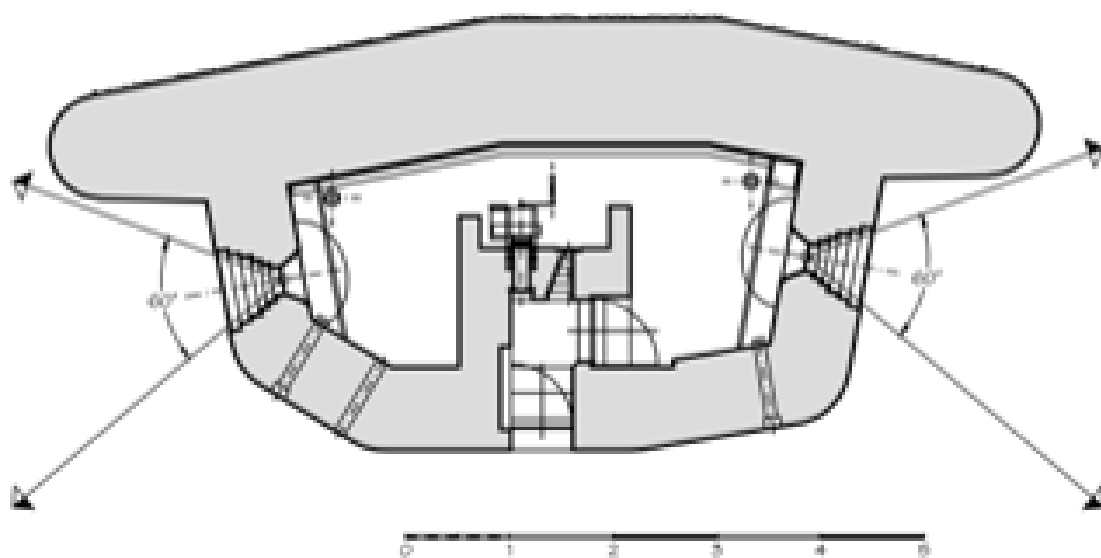
Obrázek 27 - D-31/62/A-220Z (plánový nákres)
