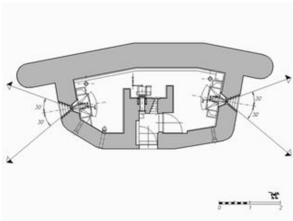
Obrázek 25 - Objekt D-31/63/A-200 (plánový nákres)
