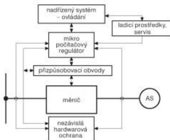
Obr. 14 Příklad použití měniče v regulační části pohonu 25
