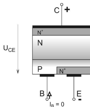
Obr. 4 Schéma bipolárního tranzistoru NPN v blokovacím stavu 4
