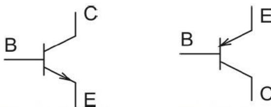
Obr. 3 Bipolární tranzistor NPN a PNP
