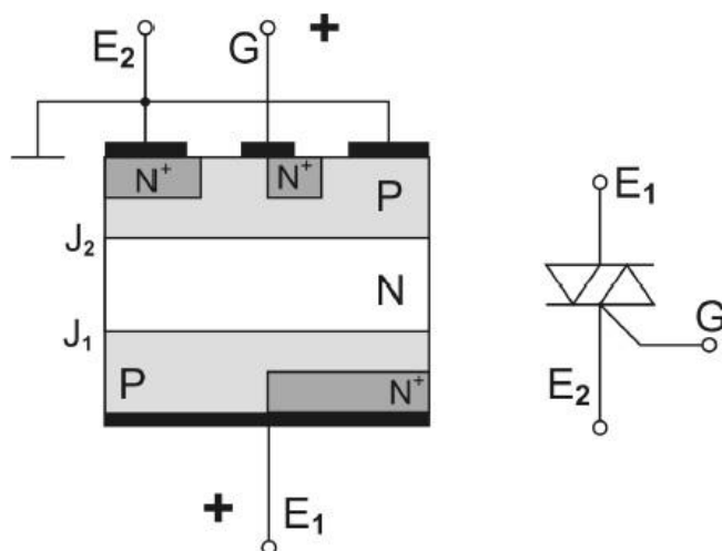
Obr. 12 Struktura a schematická značka triaku 12
