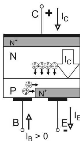
Obr. 5 Schéma bipolárního tranzistoru v sepnutém stavu 5
