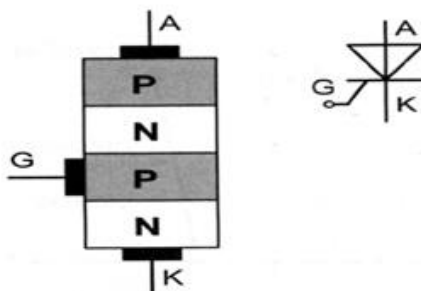
Obr. 6 Struktura a schematická značka tyristoru 6
