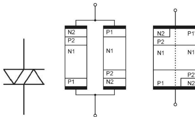
Obr. 11 Schematická značka a struktura diaku 11
