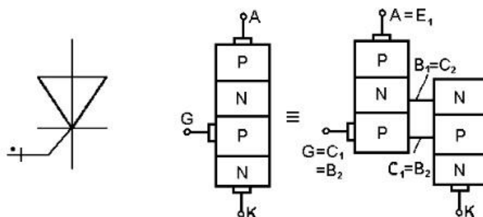
Obr. 7 Schematická značka a analogie dvou tranzistorů 7
