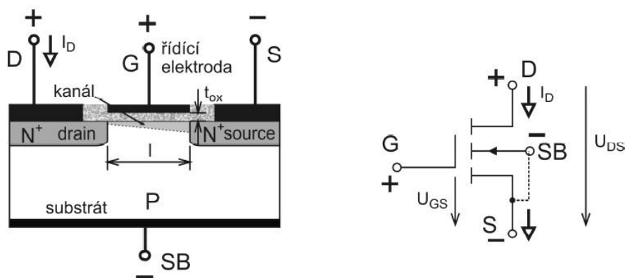
Obr. 10 Struktura a schematická značka tranzistoru MOSFET 10
