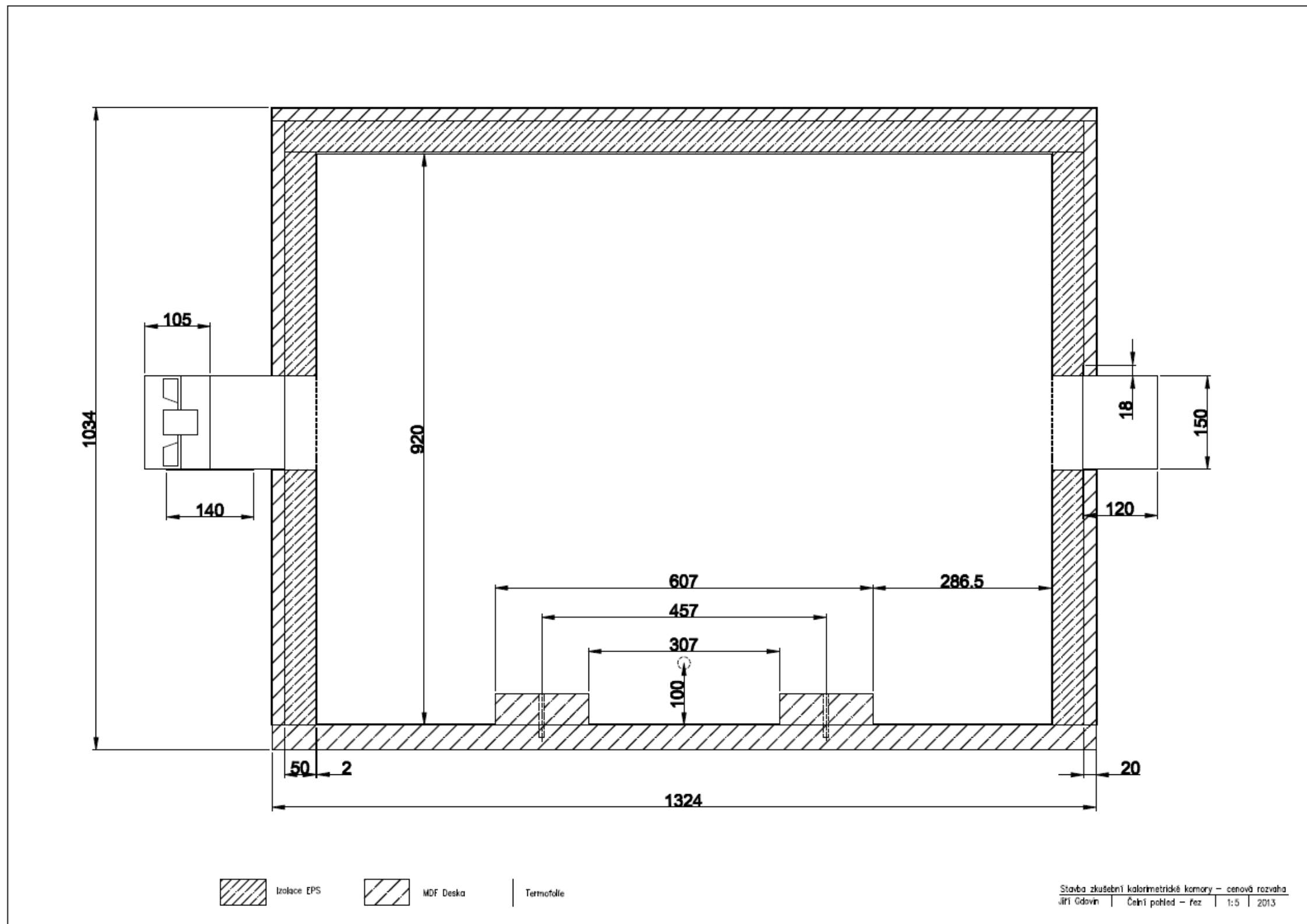
Obr. 25 – Kalorimetrická komora – čelní pohled v řezu
