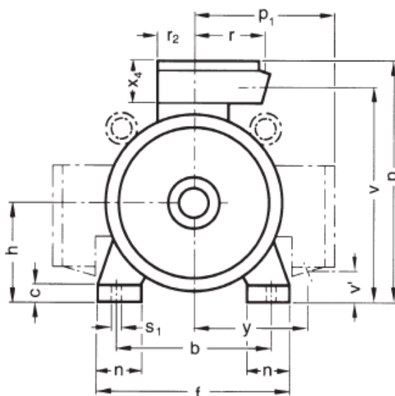
Obr. 20 - Rozměry elektrického motoru typ 280M – čelní pohled [9]
