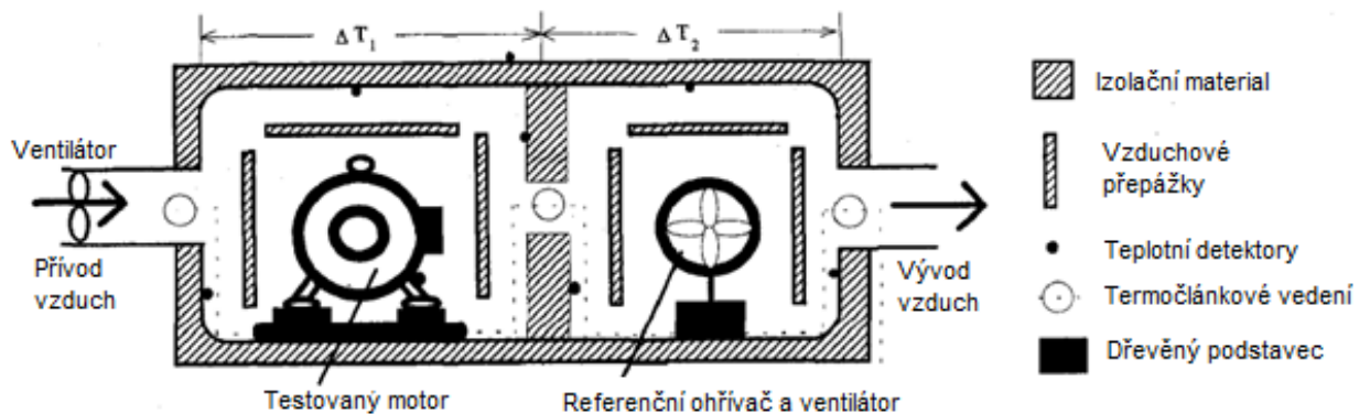
Obr. 2: Příklad konstrukce dvoukomorového kalorimetru s testovaným motorem a referenčním ohříváčem [1]
