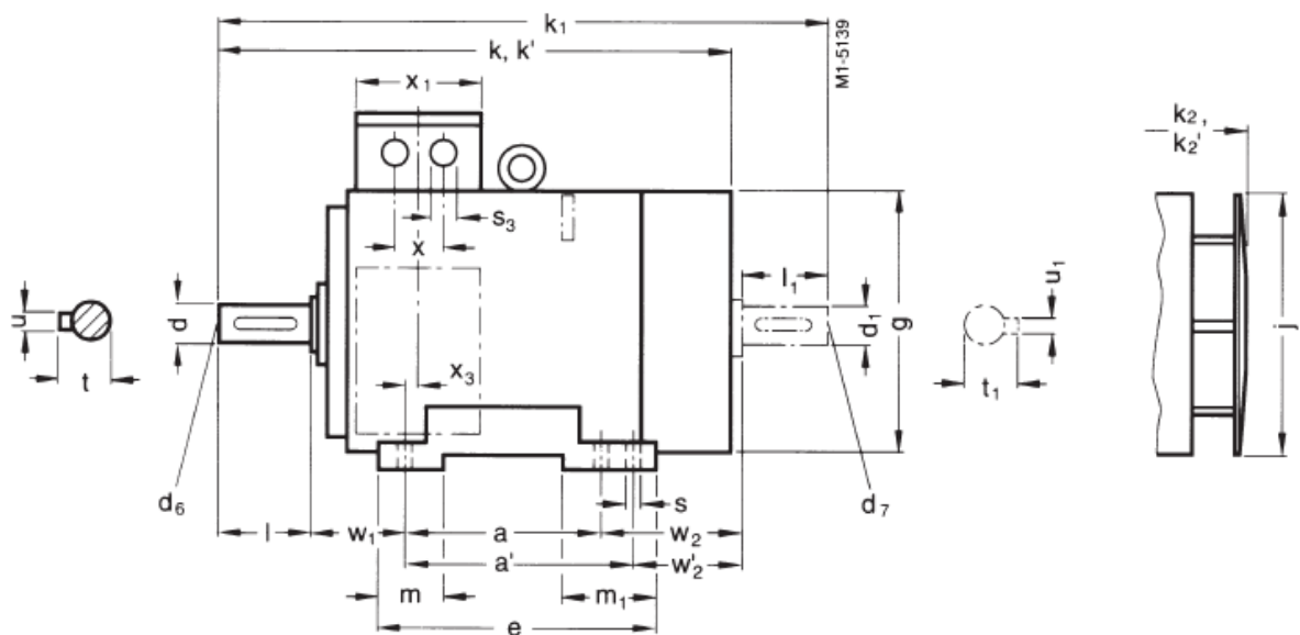
Obr. 19 – Rozměry elektrického motoru typ 280M – boční pohled [9]
