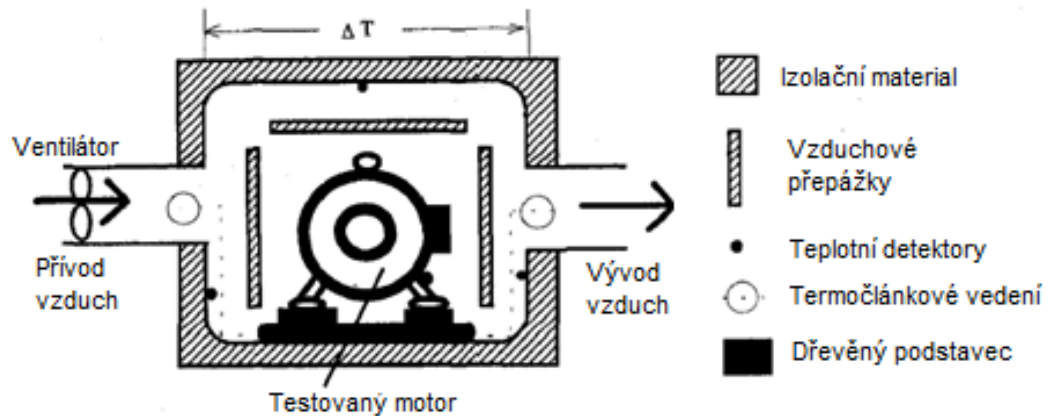
Obr. 1 Příklad konstrukce jednokomorového kalorimetru s testovaným motorem [1]
