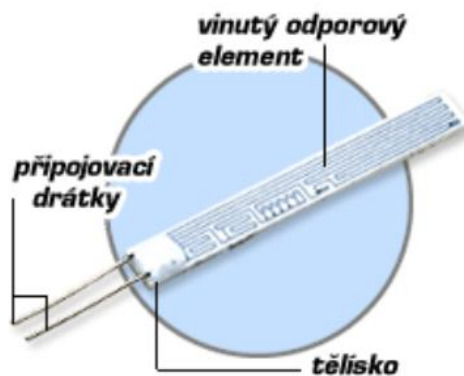
Obr. 15 – Typické provedení odporového snímače [8]
