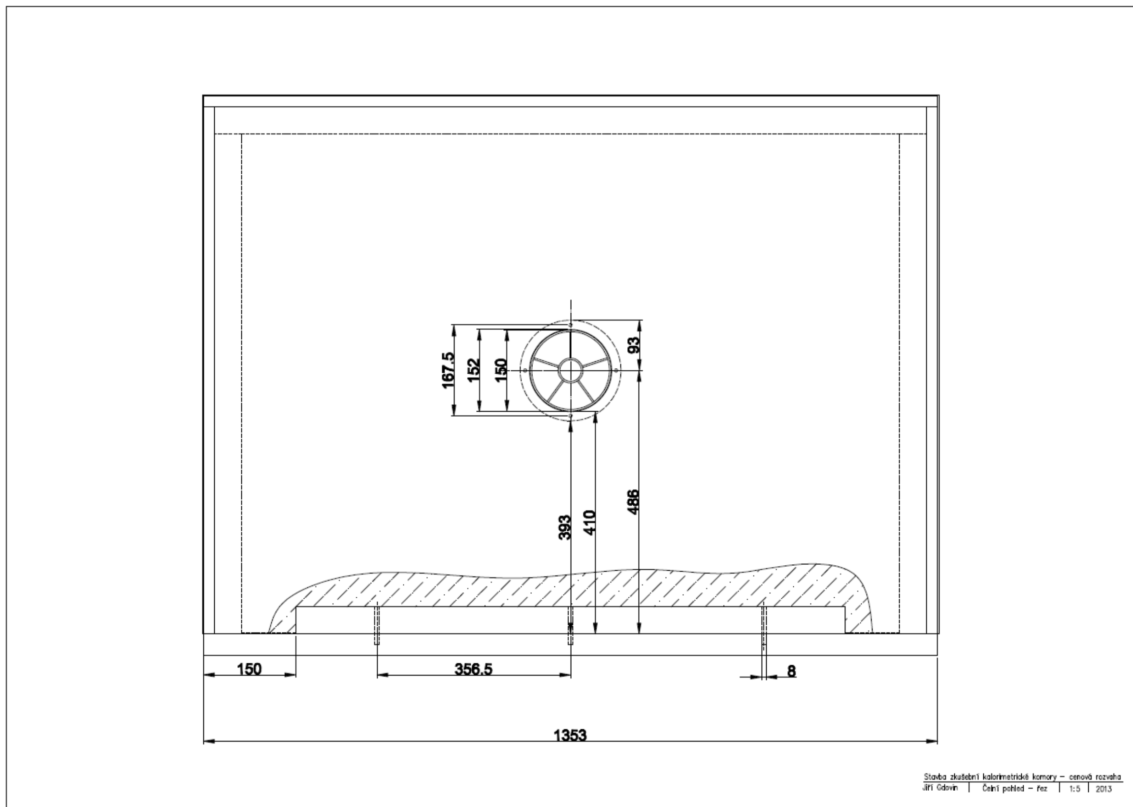
Obr. 26 – Kalorimetrická komora – boční pohled
