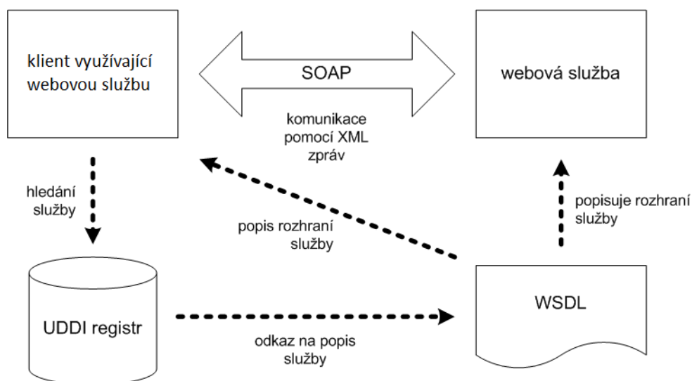
Obrázek 3.2: Vztah tří základních technologií (SOAP, WSDL a UDDI) webových služeb[10]
