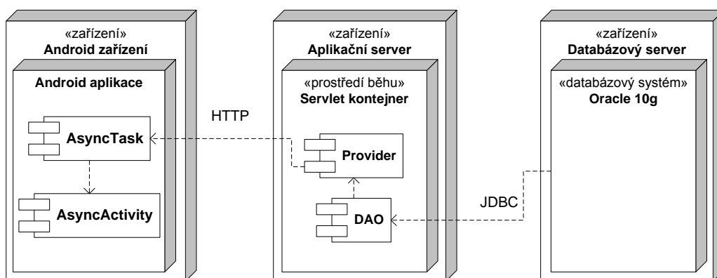
Obrázek 3.1: Diagram nasazení
