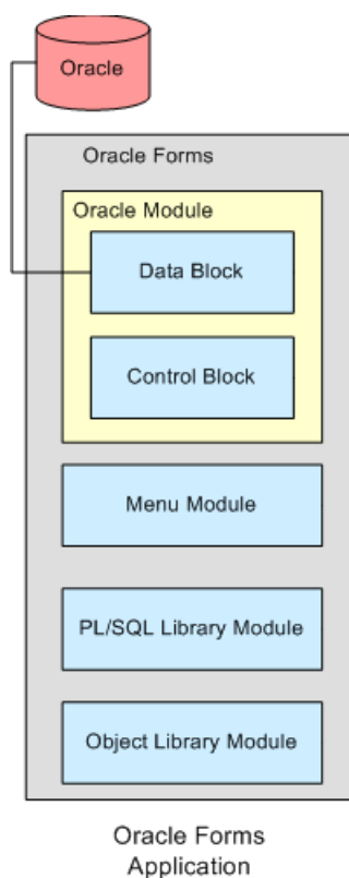
Obrázek 2.4: Komponenty Oracle Forms aplikace[20]
