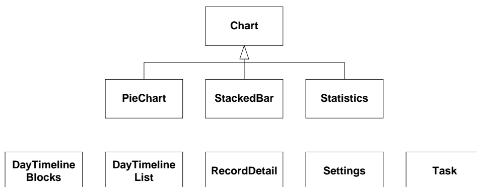
Obrázek 6.2: UML diagram tříd pro aktivity aplikace
