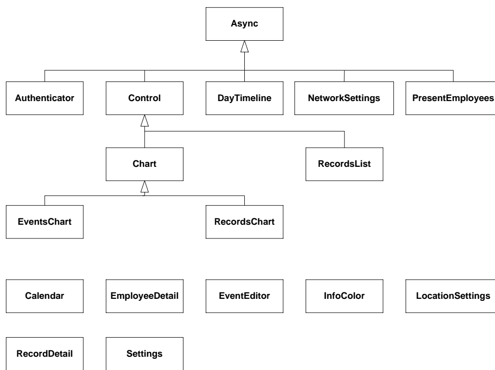
Obrázek 6.1: UML diagram tříd pro aktivity aplikace
