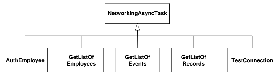
Obrázek 6.3: UML diagram tříd pro AsyncTask třídy použité v aplikaci
